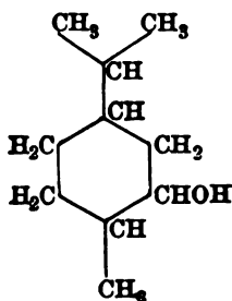
Carvomenthol.
